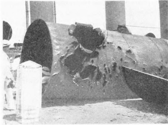
Разбитая снарядомъ труба.
