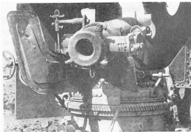
12-сантиметровая пушка Канэ.
