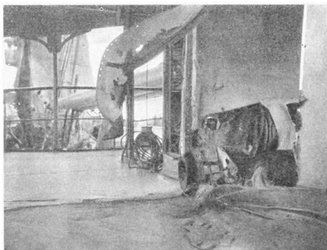
Разрушеніе мостика 12-дюймовымъ снарядомъ.
