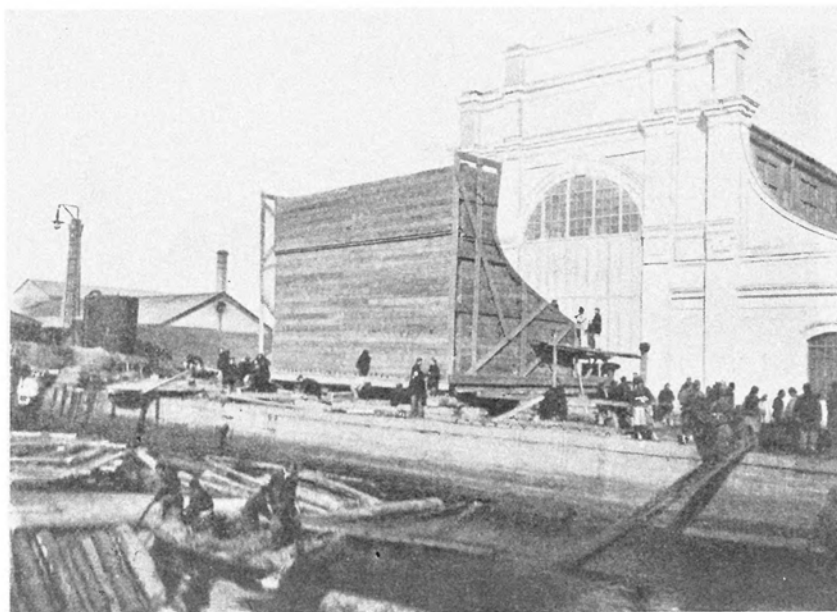
Готовый кессонъ на берегу въ Портъ-Артурѣ.
